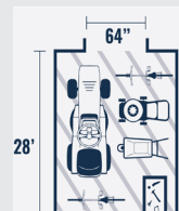
12'x28'
